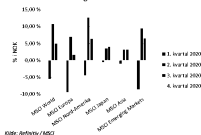
Utviklingen i MSCI indekser
