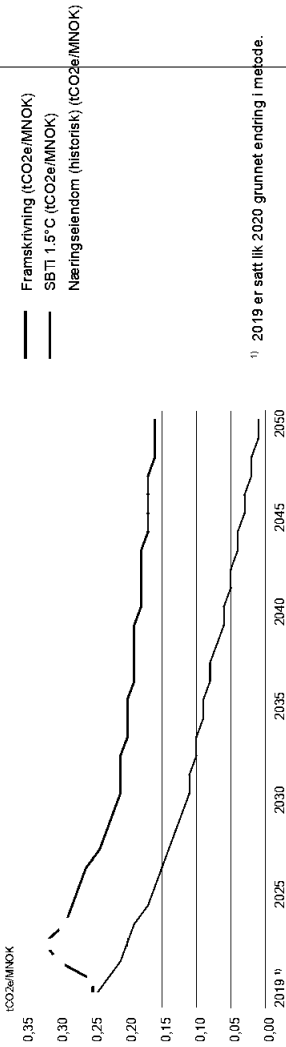
FIG. 14 Utslippsintensitet
