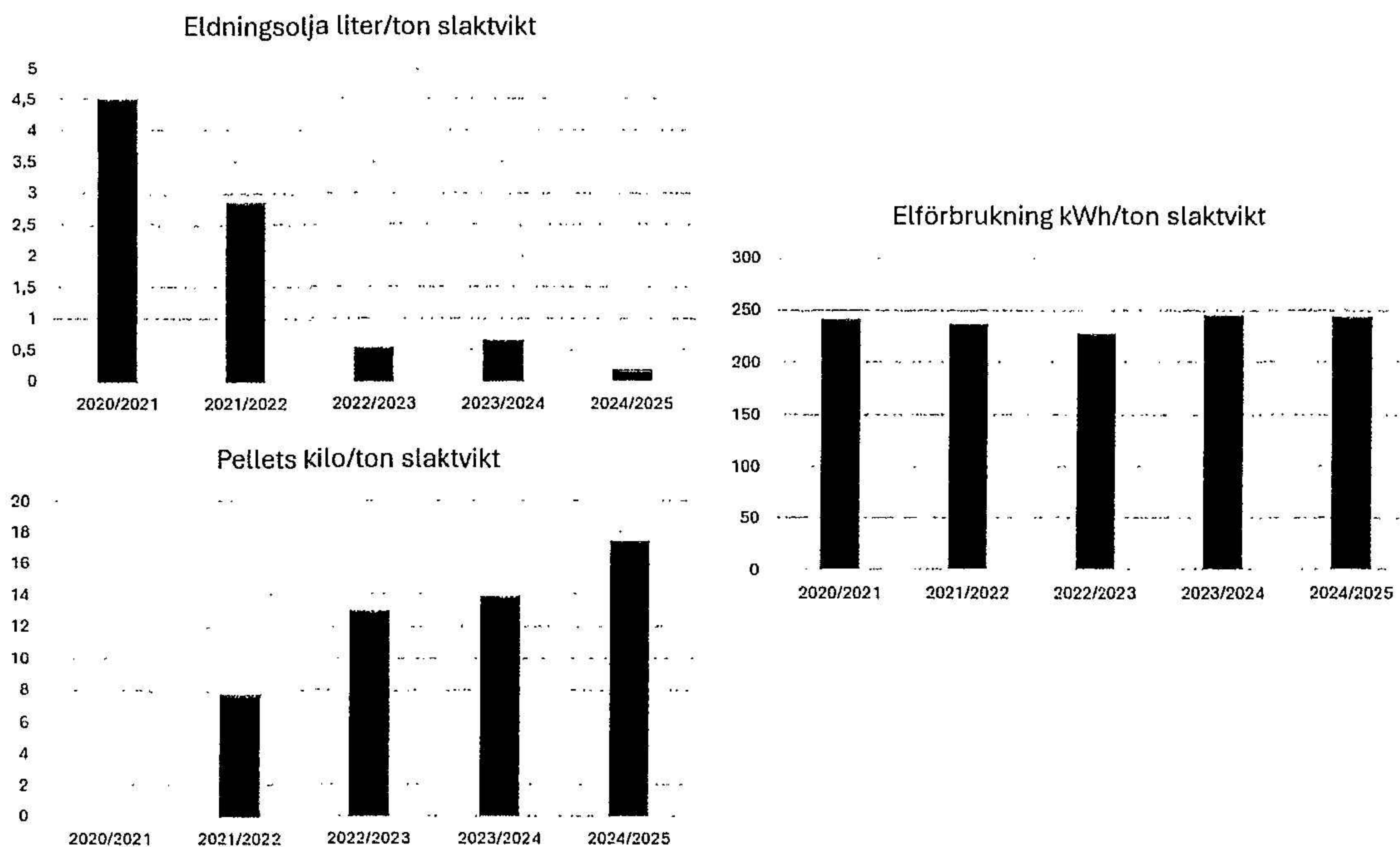
Figur 5. Förbrukning av eldningsolja, pellet och el för verksamhetsåren 2020/2021 till 2024/2025.
