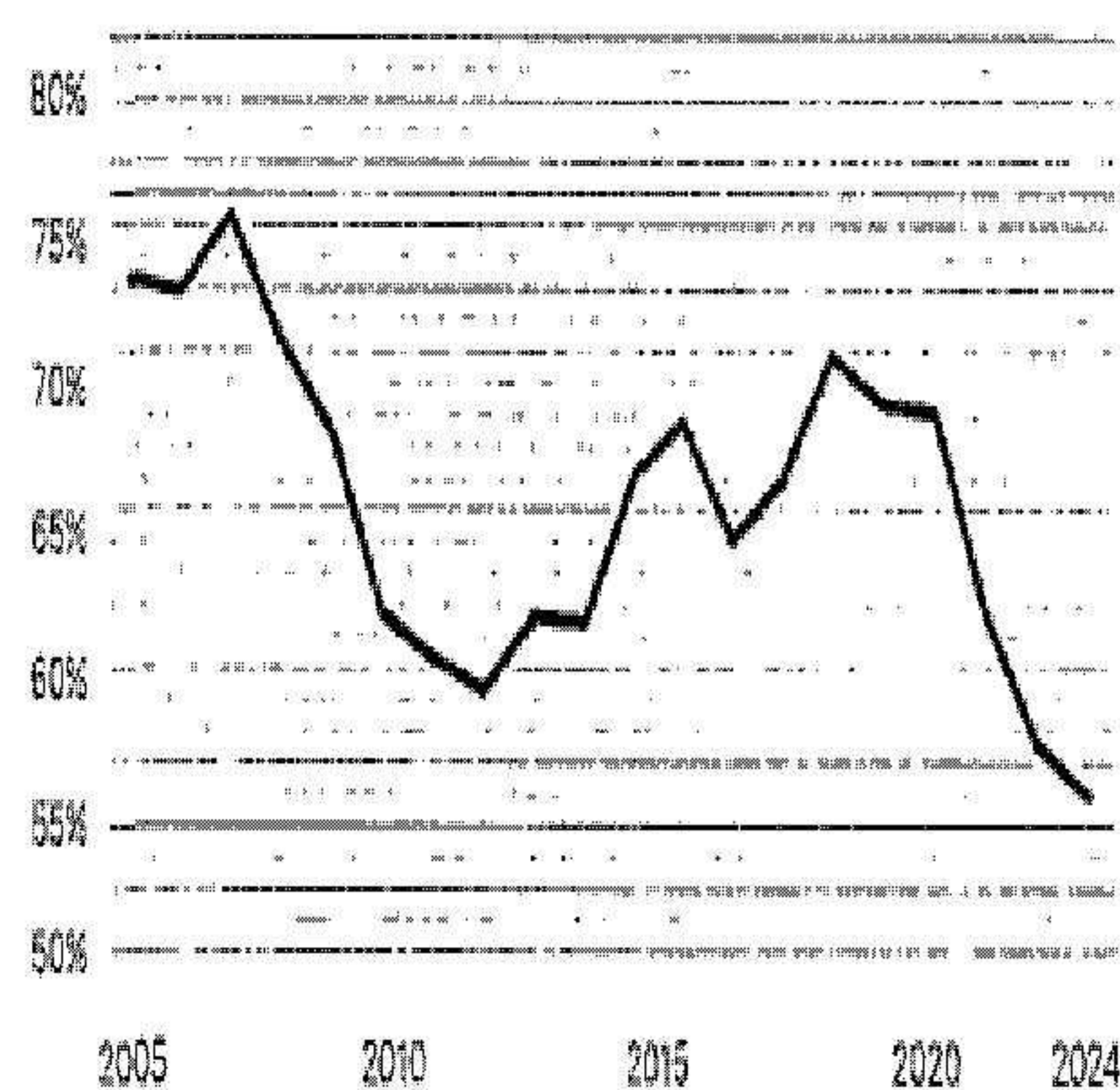
Fastigheternas belåningsgrad, %
